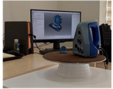
ARTEC 3D SPACE SPIDER 3 BOYUTLU TARAYICI
